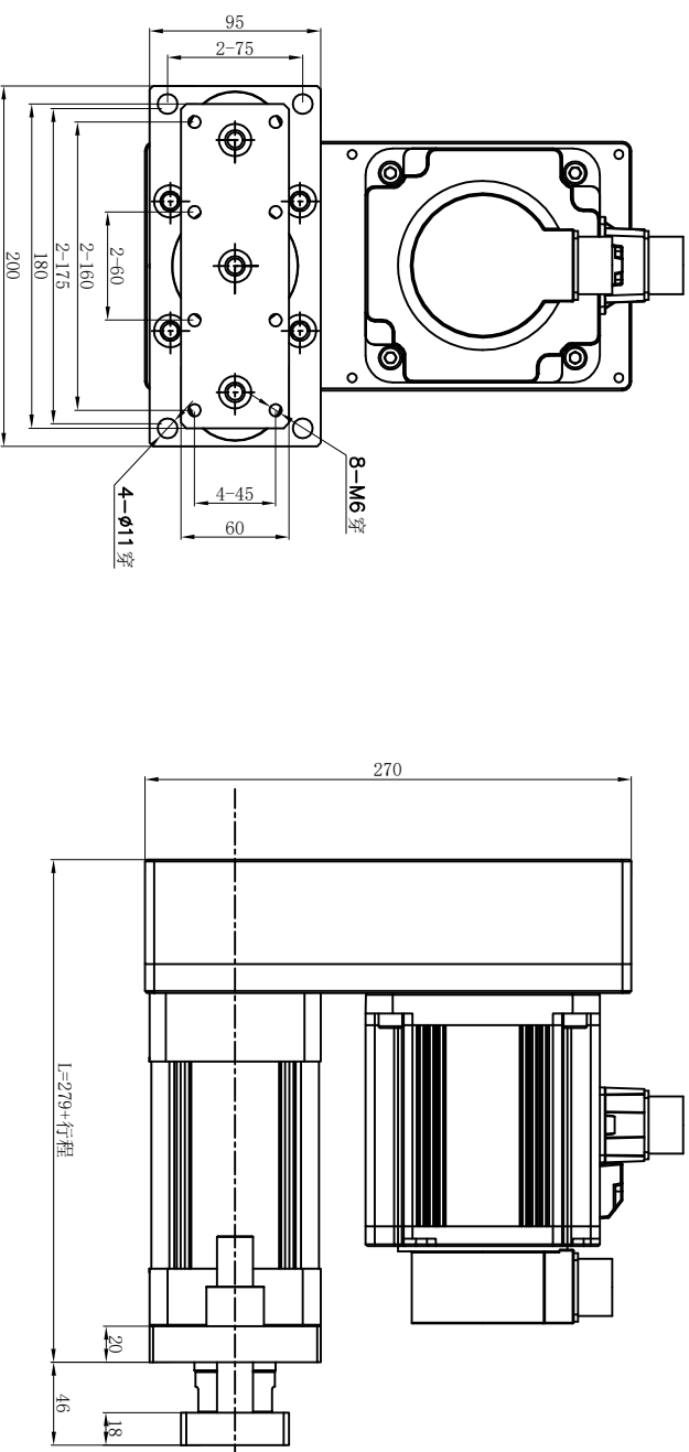
XL1-80系列折返式 前导向安装 (FG) 尺寸图
